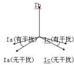
图 11 投影法 图 12 一字排列避雷器 图 13 AC 相受 B 相影响
