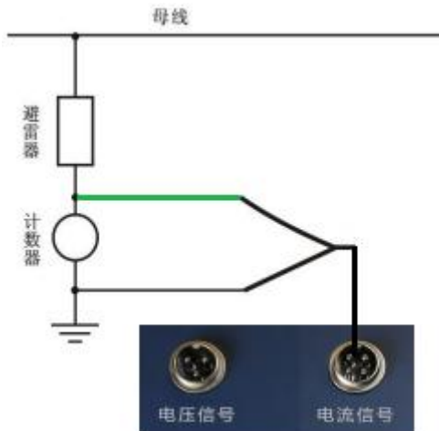
图 4 无线模式(测试相序: B)测量接线示意图
