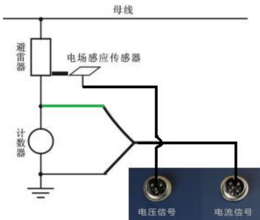
图 5 感应模式测试接线示意图
