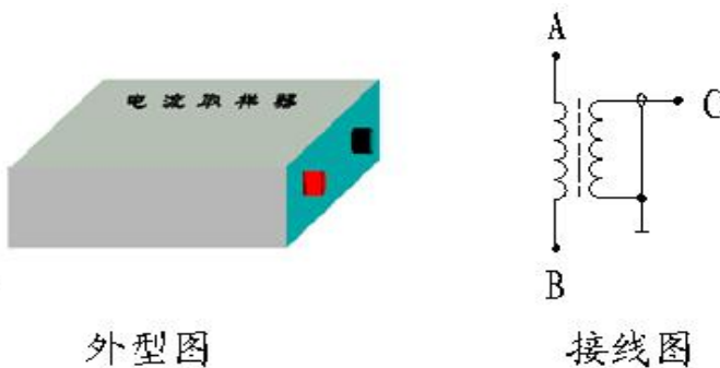
电流取样器外型及接线图
