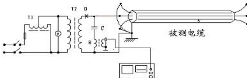
直闪法电流取样接线图
