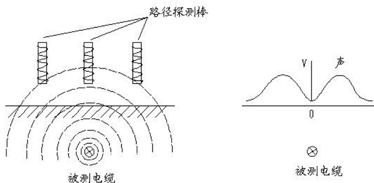
电缆路径探测原理图
