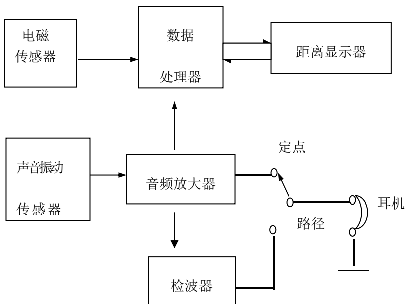
图 2 原理框图
