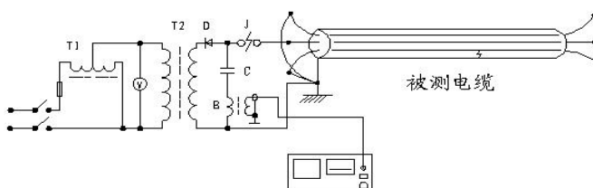
冲闪法电流取样接线图
