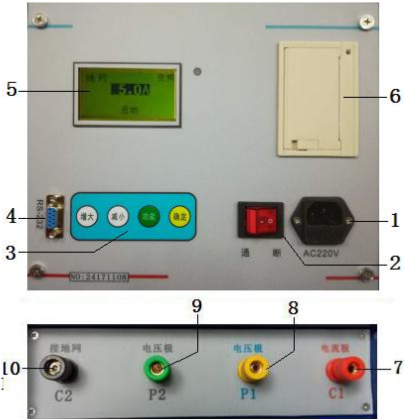
图 2 面板示意图
