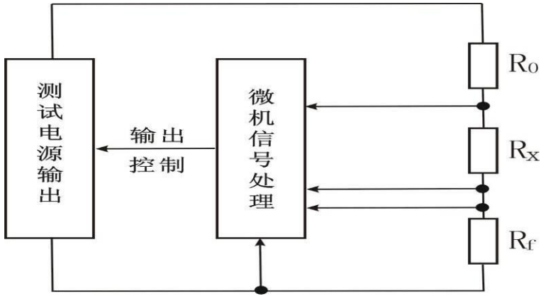
图 1 测量原理示意图
