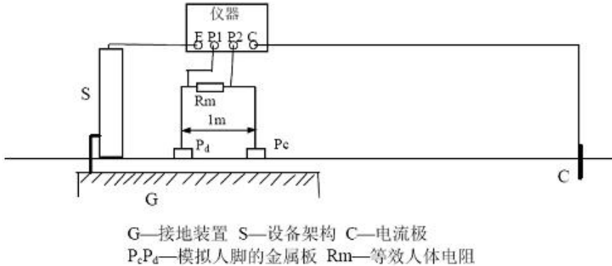
图6 跨步电压测量接线图
