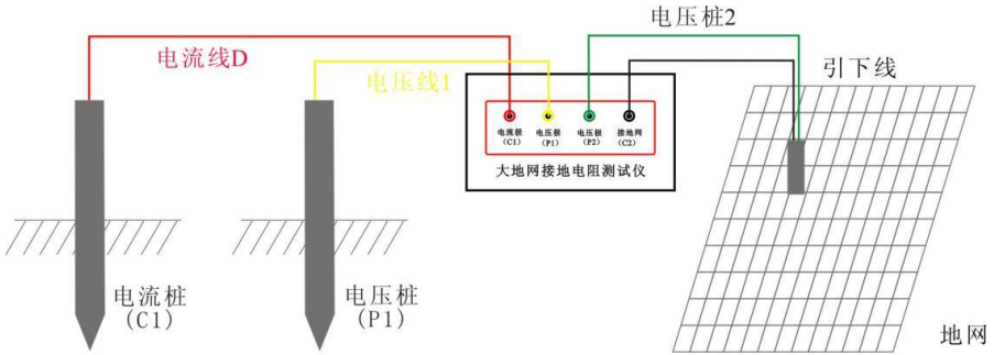
图 4 四极法测量接线图
