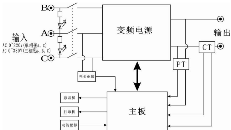
图 1 仪器内部结构及基本原理
