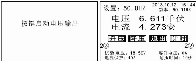
图 9：测量准备界面
