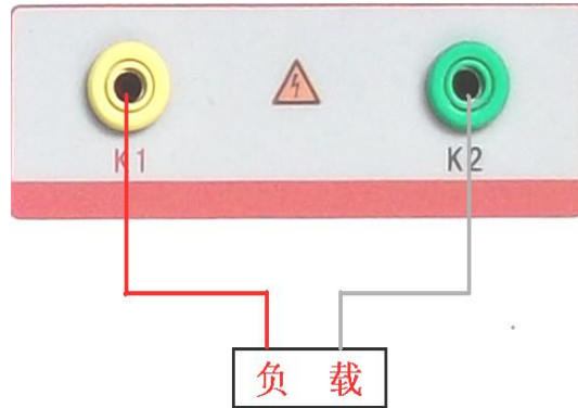
图 35, CT 二次负荷接线图
