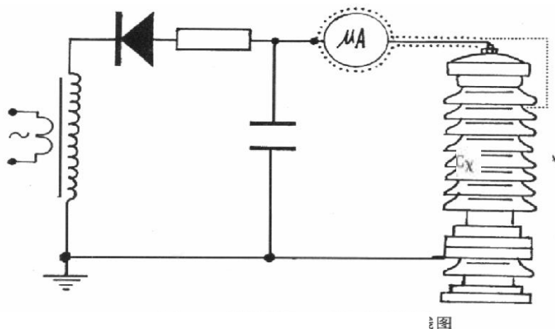
图 6 排除试品 CX 表面影响接线图
